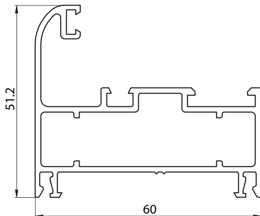
6055 - MARCO PAÑO FIJO Y VENTANA DE ABRIR PESO: 1,037 Kg/m
