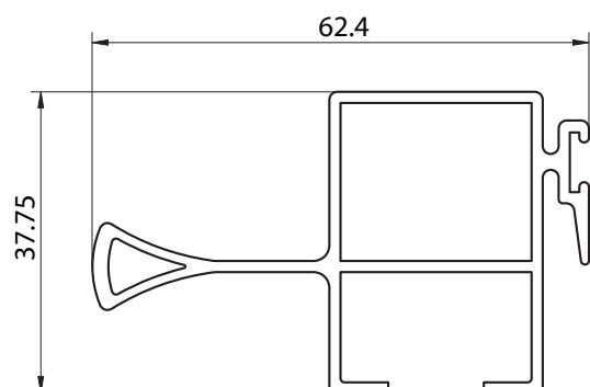
6208 - PARANTE CENTRAL CON TIRADOR HOJA PARA VIDRIO SIMLE PUERTA CORREDIZA - PESO: 0,813 kg/m
