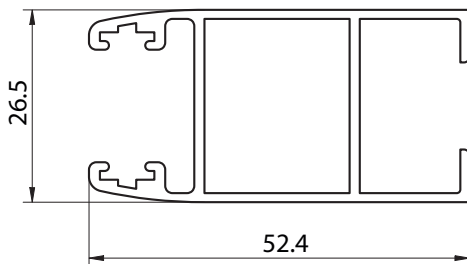
6203 - PARANTE LATERAL HOJA VIDRIO SIMPLE VENTANA Y PUERTA CORREDIZA - PESO: 0,651 kg/m
