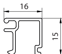
108 - CONTRAVIDRIO HERRERO - PESO: 0.355 KG x Mts.
