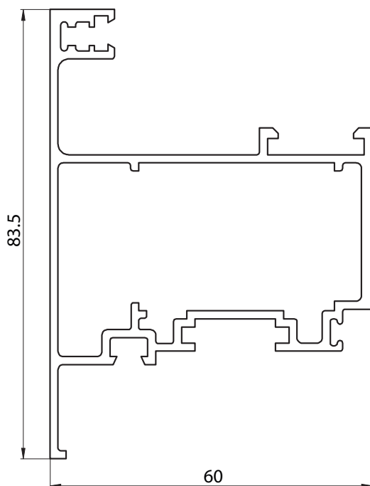
6058 - HOJA RECTA VENTANA DESPLAZABLE PESO: 1,345 Kg/m
