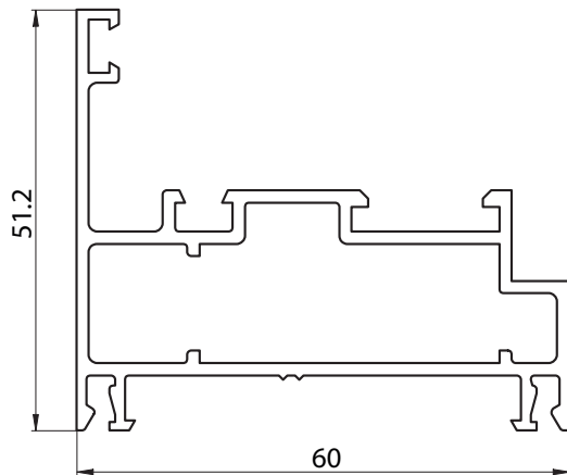
6051 - MARCO VENTANA DE ABRIR - PESO: 0,986 Kg/m
