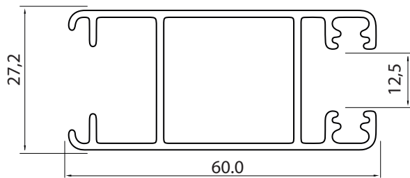
53 - PARANTE LATERAL REFORZADO HOJA CORTE A 90 PESO: 0.645 KG x Mts.
