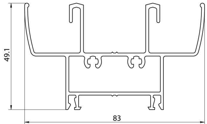
6200 - UMBRAL Y DINTEL MARCO VENTANA Y PUERTA CORREDIZA - PESO: 1,266 kg/m
