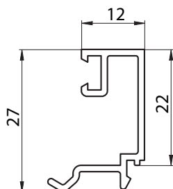
6049 - CONTRAVIDRIO RECTO LADO EXT. PUERTA DE REBATIR - PESO: 0,232 Kg/m
