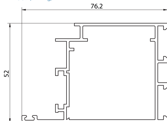
6214 - JAMBAS Y CABEZAL HOJA PUERTA DE REBATIR PESO: 1,088 kg/m
