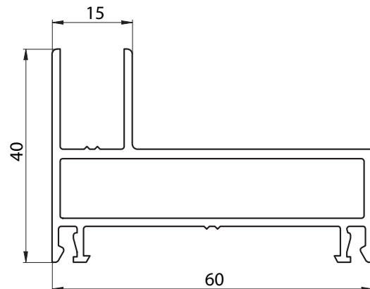
6036 - JAMBAS DE MARCO - PESO: 0,891 Kg/m
