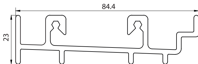
17 - MARCO DE ALTO TRÁNSITO- PESO: 1.100 KG x Mts.
