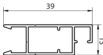
105 - HOJA MOSQUITERO - PESO: 0.278 KG x Mts.
