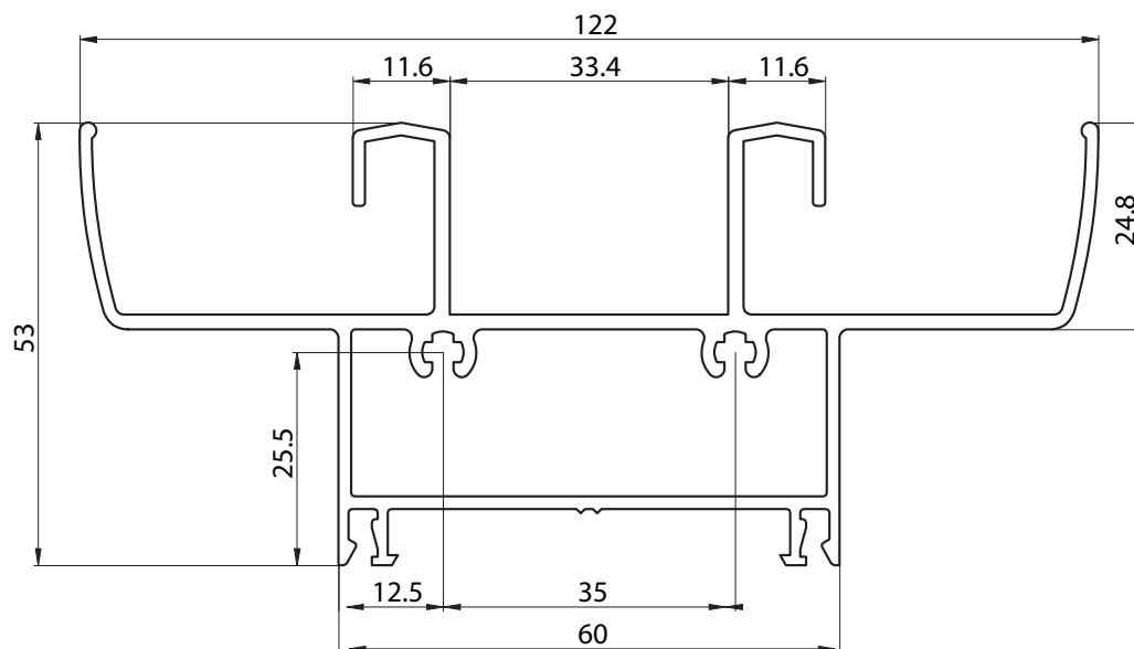
6037 - UMBRAL Y DINTEL DE MARCO - PESO: 1,744 Kg/m
