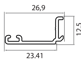
45 - TAPA JUNTA - PESO: 0.144 KG x Mts.
