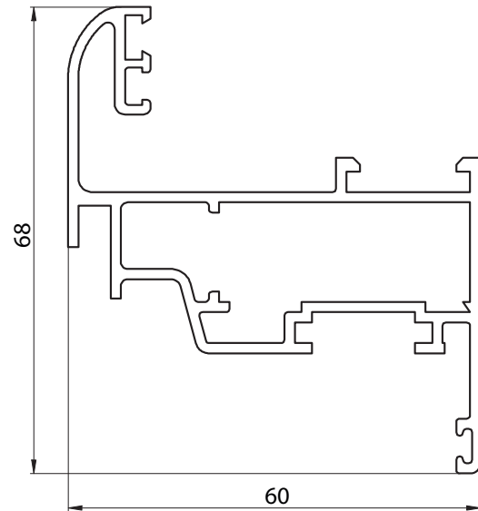
6052 - HOJA CURVA VENTANA DE ABRIR PESO: 1,139 Kg/m
