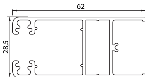
6909 - HOJA DVH CORREDIZA 45° - PESO: 0,840 Kg/m
