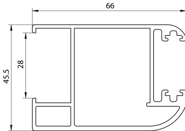
6071 - PARANTE LATERAL CORREDIZA P/DVH PESO: 1,334 Kg/m
