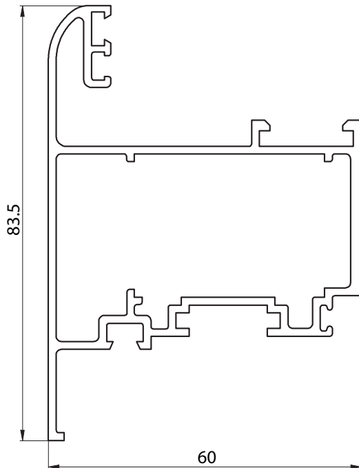
6056 - HOJA CURVA VENTANA DESPLAZABLE PESO: 1,337 Kg/m
