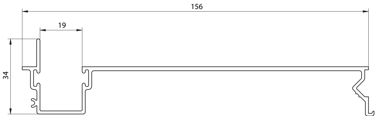
6065 - GUÍA DE CORTINA BARRIO - PESO: 1,088 Kg/m
