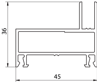
6201 - JAMBAS DE MARCO VENTANA Y PUERTA CORREDIZA - PESO: 0,664 kg/m
