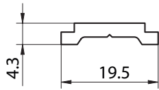
5989 - VARILLA DE ACCIONAMIENTO CIERRE VENTANA DE ABRIR Y PUERTA DE REBATIR - PESO: 0,141 kg/m
