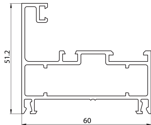
6059 - MARCO RECTO PAÑO FIJO Y VENTANA DE ABRIR - PESO: 1,053 Kg/m
