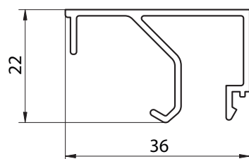
6212 - CONTRAVIDRIO 36 MM. - PESO: 0,316 kg/m
