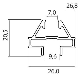
31 - PERFIL LATERAL VIDRIO REPARTIDO PESO: 0.264 KG x Mts.
