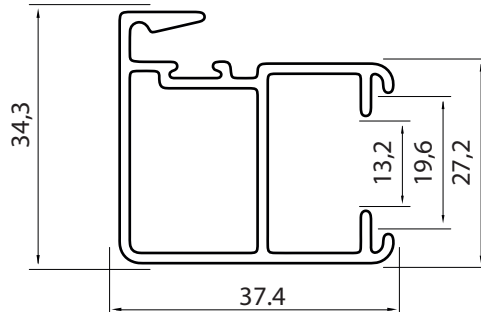
54 - PARANTE CENTRAL REFORZADO PESO: 0.498 KG x Mts.
