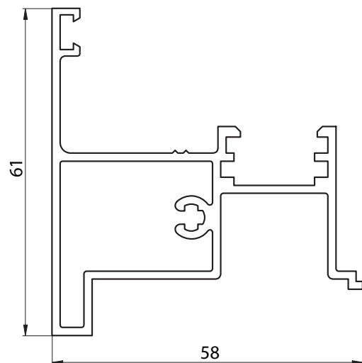
6044 - ENCUENTRO CENTRAL PUERTA DE REBATIR PESO: 1,037 Kg/m
