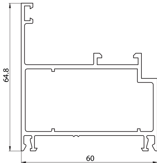
6040 - MARCO DE PUERTA REBATIR COPLANAR PESO: 1,180 Kg/m
