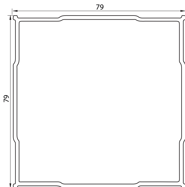
185 - COLUMNA ACOUPLE RECTO - PESO: 1,339 KG x Mts.
