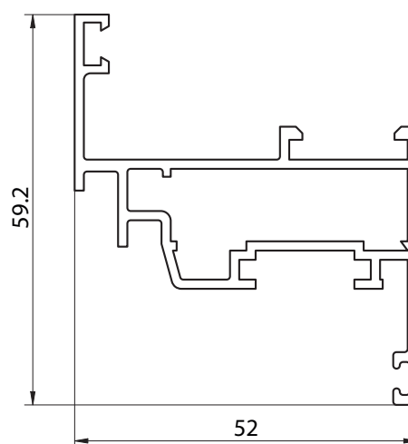
6211 - HOJA VENTANA DE ABRIR CON CÁMARA COMPENSADORA - PESO: 0,848 kg/m
