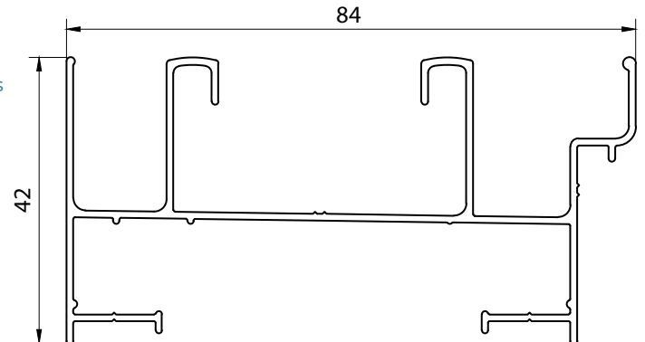
101 - MARCO DE CORREDIZA - PESO: 0.742 KG x Mts.
