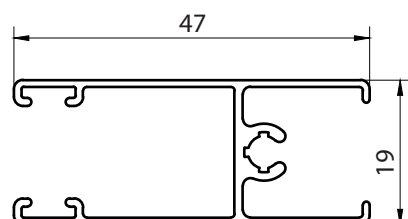
102 - CABEZAL Y ZÓCALO DE HOJA PESO: 0.443 KG x Mts.
