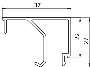
6045 - CONTRAVIDRIO RECTO P/VIDRIO SIMPLE PESO: 0,351 Kg/m
