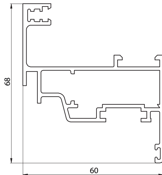
6054 - HOJA RECTA VENTANA DE ABRIR PESO: 1,148 Kg/m
