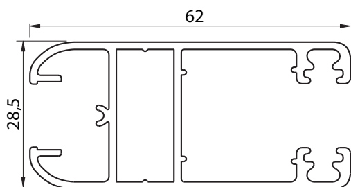
6908 - HOJA VIDRIO SIMPLE CORREDIZA 45° PESO: 0,894 Kg/m
