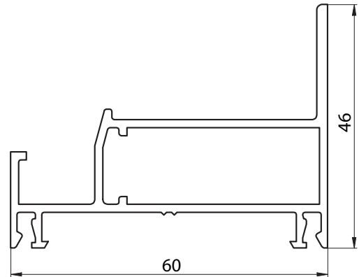
6057 - MARCO VENTANA DESPLAZABLE PESO: 0,837 Kg/m
