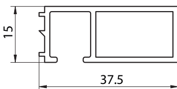
6205 - PREMARCO - PESO: 0,410 kg/m
