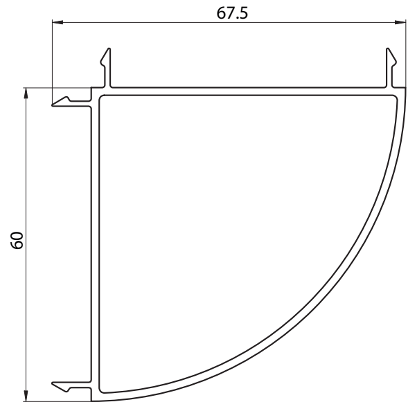
6069 - ACOPLE A 90 GRADOS - PESO: 0,937 Kg/m
