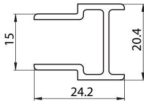
5965 - ENCUENTRO CENTRAL CORREDIZA DE 4 HOJAS PESO: 0,288 Kg/m
