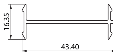
6213 - PERFIL DE ACOPLE - PESO: 0,257 kg/m
