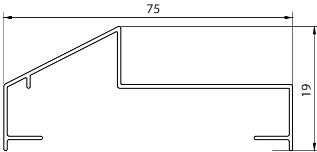
48 - MARCO PUERTA PLACA 45 - PESO: 0.355 KG x Mts.
