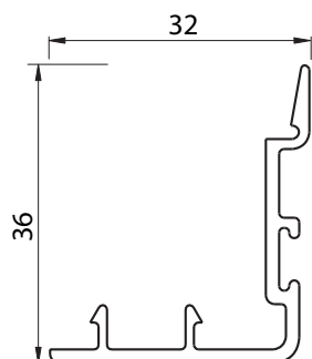
6907 - COMPLEENTO PARANTE CENTRAL CORREDIZA 45° - PESO: 0,338 Kg/m
