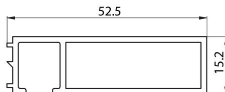
6066 - PREMARCO - PESO: 0,545 Kg/m
