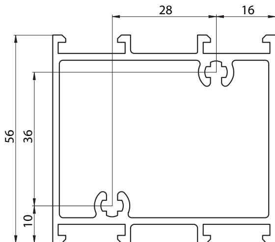
6042 - MARCO PUERTA DE REBATIR - PESO: 1,399 Kg/m
