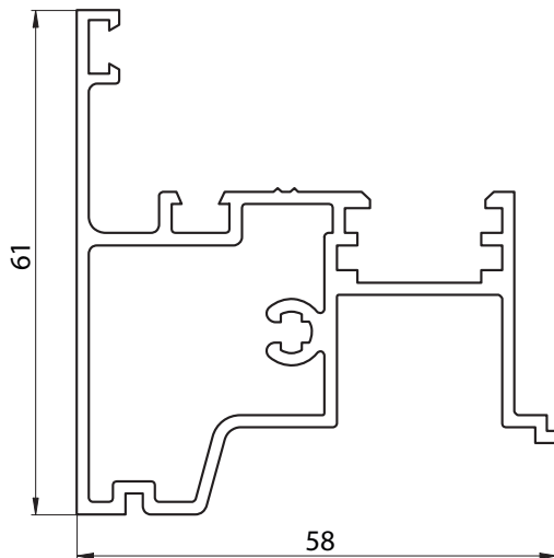
6053 - ENCUENTRO CENTRAL VENTANA DE ABRIR PESO: 1,094 Kg/m
