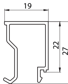
6046 - CONTRAVIDRIO RECTO P/DVH - PESO: 0,259 Kg/m
