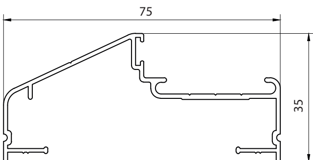
39 - MARCO PUERTA 36 - PESO: 0.536 KG x Mts.
