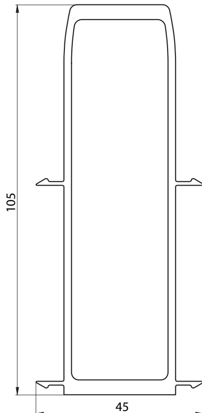
6078 - PERFIL DE ACOPLE REFORZADO PESO: 1,758 Kg/m
