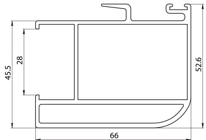
6072 - PARANTE CENTRAL CORREDIZA P/DVH PESO: 1,466 Kg/m
