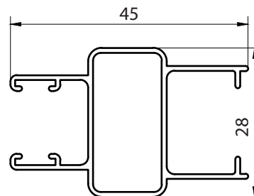
103 - PARANTE LATERAL HOJA CORREDIZA PESO: 0.454 KG x Mts.
