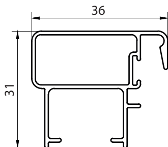
107 - PAÑO FIJO HERRERO - PESO: 0.650 KG x Mts.
