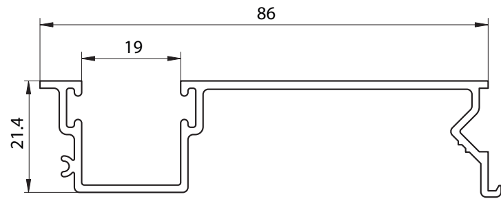
6064 - GUÍA DE CORTINA COMÚN - PESO: 0,672 Kg/m
