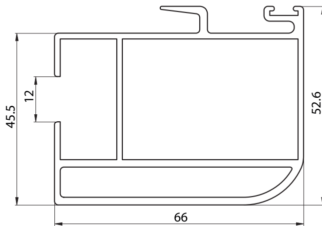
6035 - PARANTE CENTRAL CORREDIZA - PESO: 1,531 Kg/m
