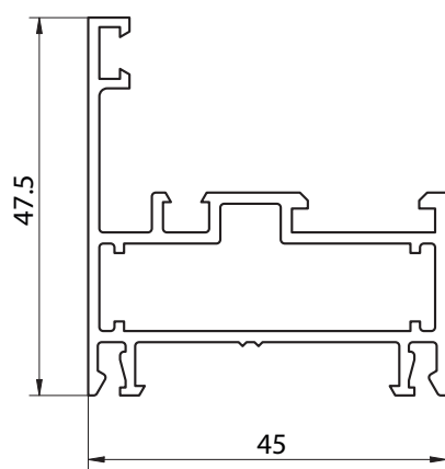
6212 - CONTRAVIDRIO 36 MM. - PESO: 0,316 kg/m
