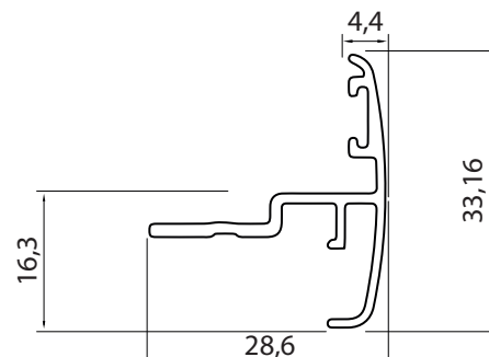
37 - DOBLE CONTACTO PUERTA 25 MM PESO: 0.268 KG x Mts.
