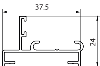
32 - PESO: 0.274 KG x Mts.
