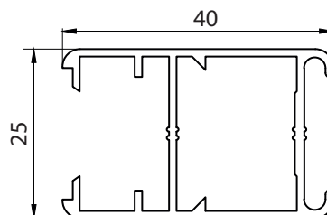
178 - PARANTE POSTIGÓN CHICO - PESO: 0.464 KG x Mts.
