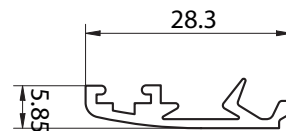
6206 - TAPA PREMARCO - PESO: 0,181 kg/m
