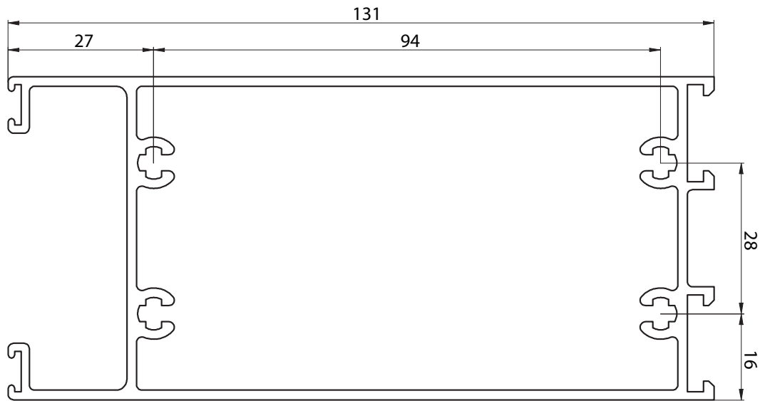
6045 - CONTRAVIDRIO RECTO P/VIDRIO SIMPLE PESO: 0,351 Kg/m
