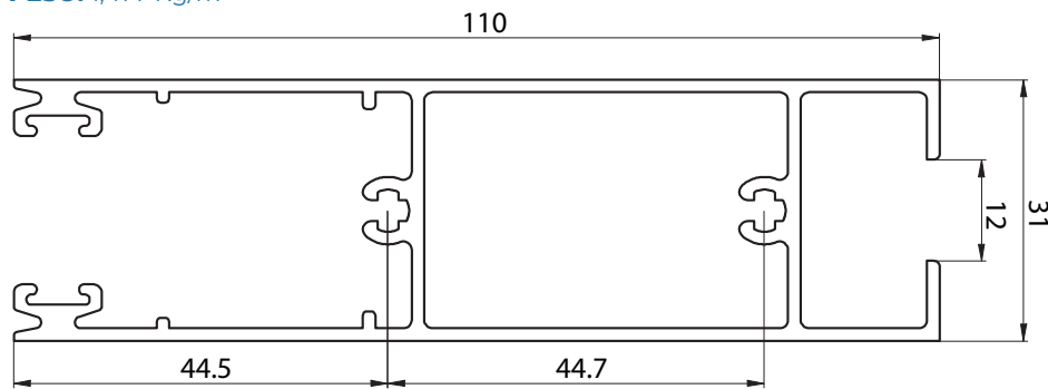
6062 - ZÓCALO ALTO PUERTA CORREDIZA PESO: 1,477 Kg/m
