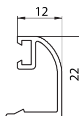
6050 - CONTRAVIDRIO CURVO LADO EXT. PUERTA DE REBATIR - PESO: 0,192 Kg/m
