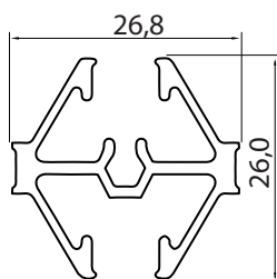
30 - PERFIL CENTRAL VIDRIO REPARTIDO PESO: 0.383 KG x Mts.
