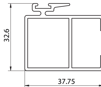
6207 - PARANTE CENTRAL HOJA PARA VIDRIO SIMPLE PUERTA Y VENTANA CORREDIZA - PESO: 0,613 kg/m
