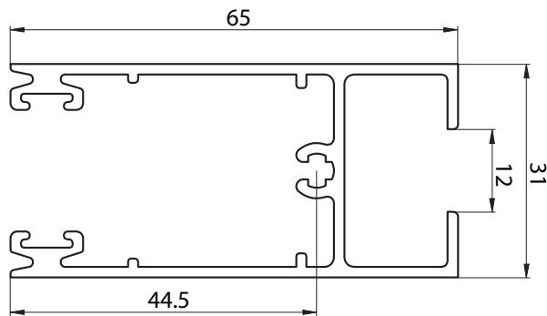
6061 - ZÓCALO Y CABEZAL VENTANA CORREDIZA PESO: 0,942 Kg/m
