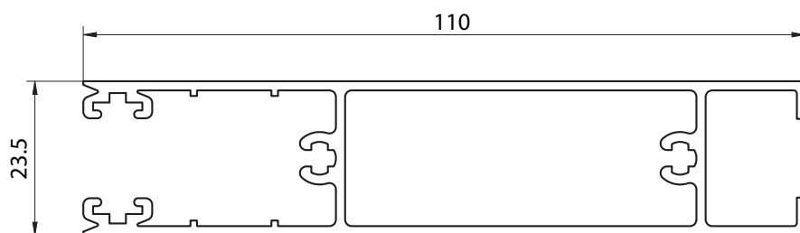
6209 - ZÓCALO ALTO HOJA PARA VIDRIO SIMPLE PUERTA CORREDIZA - PESO: 1,266 kg/m
