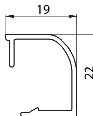
6048 - CONTRAVIDRIO CURVO P/DVH - PESO: 0,197 Kg/m
