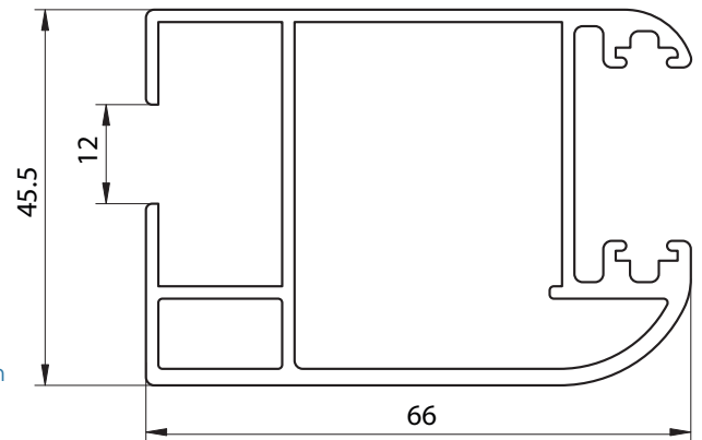
6035 - PARANTE CENTRAL CORREDIZA - PESO: 1,531 Kg/m
