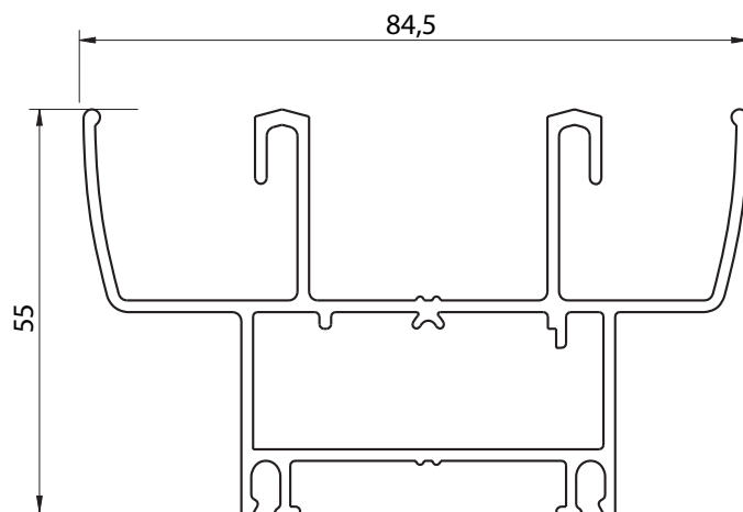
6909 - HOJA DVH CORREDIZA 45° - PESO: 0,840 Kg/m
