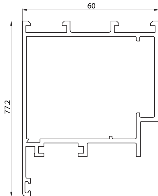
6041 - HOJA PUERTA DE REBATIR - PESO: 1,388 Kg/m
