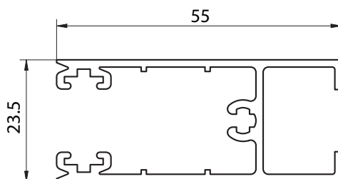
6204 - ZÓCALO Y CABEZAL DE HOJA PARA VIDRIO SIMPLE VENTANA Y PUERTA CORREDIZA PESO: 0,705 kg/m
