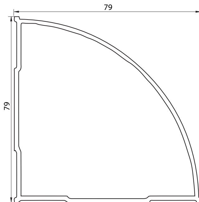
186 - COLUMNA ACOUPLE CURVO - PESO: 1,204 KG x Mts.
