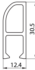
6039 - TOPE MOSQUITERO - PESO: 0,329 Kg/m
