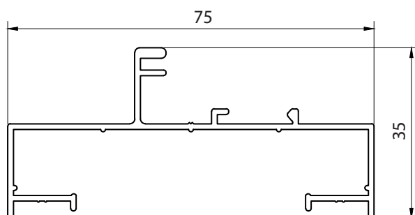
107 - PAÑO FIJO HERRERO - PESO: 0.650 KG x Mts.
