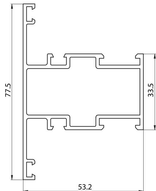
6060 - TRAVESAÑO PAÑO FIJO - PESO: 1,091 Kg/m
