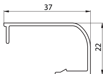
6047 - CONTRAVIDRIO CURVO P/VIDRIO SIMPLE PESO: 0,254 Kg/m
