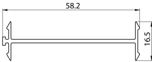
6067 - PERFIL DE ACOPLE - PESO: 0,329 Kg/m
