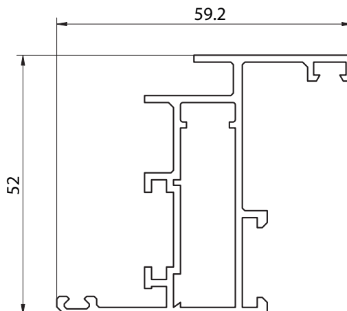
6215 - HOJA VENTANA DE ABRIR DOBLE CONTACTO/ BANDEROLA - PESO: 0,864 kg/m
