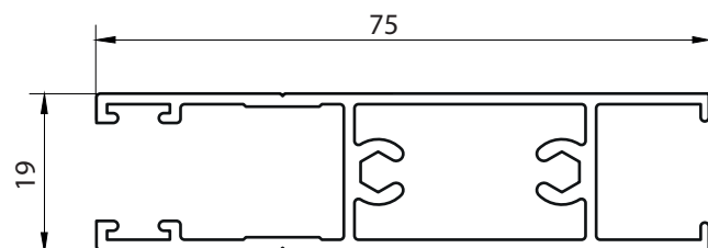
44 - ZOCALO ALTO PUERTA CORREDIZA PESO: 0.848 KG x Mts.
