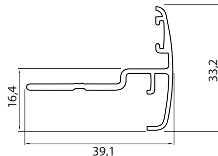
40 - DOBLE CONTACTO PUERTA 36 MM PESO: 0.311 KG x Mts.
