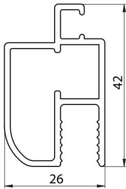
6038 - MOSQUITERO REFORZADO - PESO: 0,594 Kg/m
