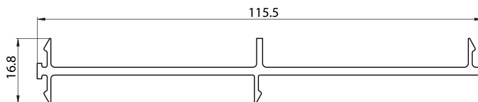
6068 - ACOUPLE 60 MM A MARCO DE 3 GUÍAS PESO: 0,753 Kg/m
