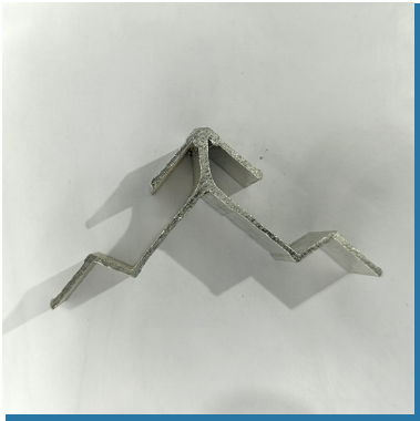
E68 ALUMINIO x50 ESCUADRA DE ARMADO PREMARCO CORTE 45º MODENA
