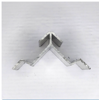
PARTE C X50 ESCUADRA DE ARMADO
