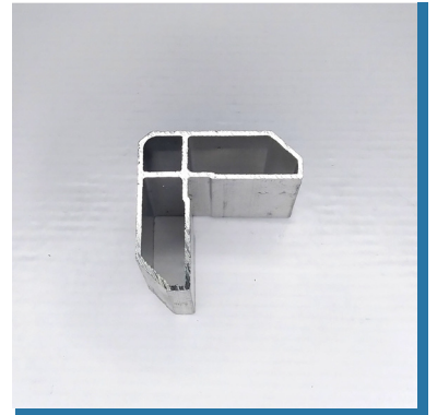
E67 x 1 ESCUADRA SUPLEMENTARIA PARA E70 MODENA
